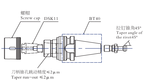
DBT40-45-DSK11-075 (命名示意图 Naming diagram)
