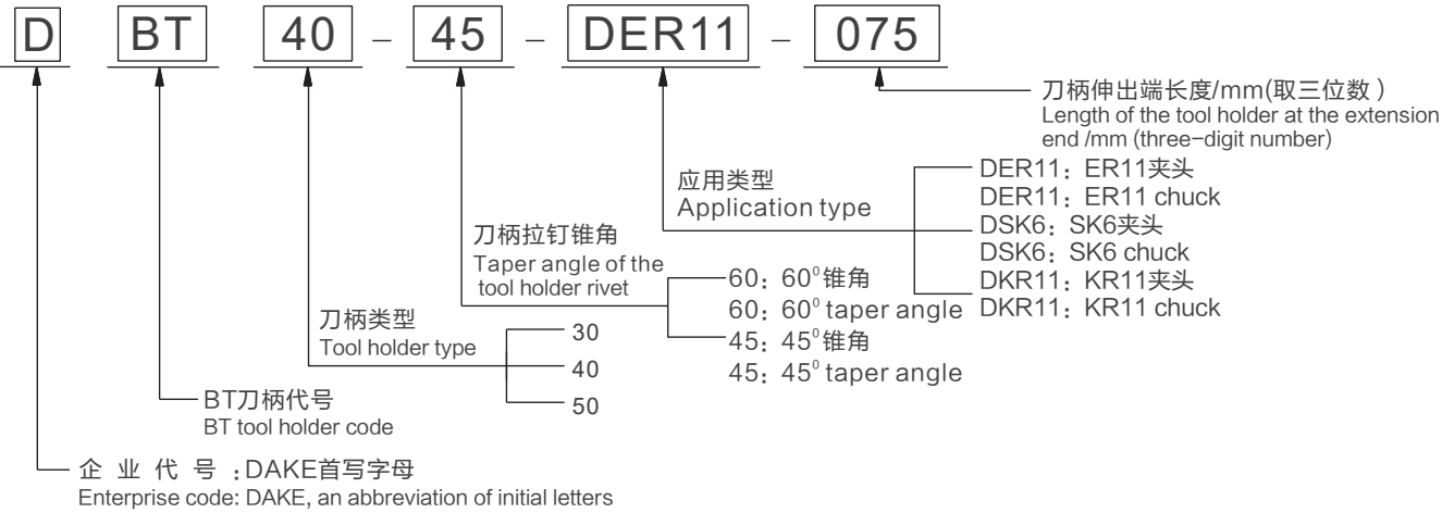
DBT40-45-DER11-075 (命名示意图 Naming diagram) DBT40-45-DER11-075 (装刀精度示意图 Tool installation precision diagram)
