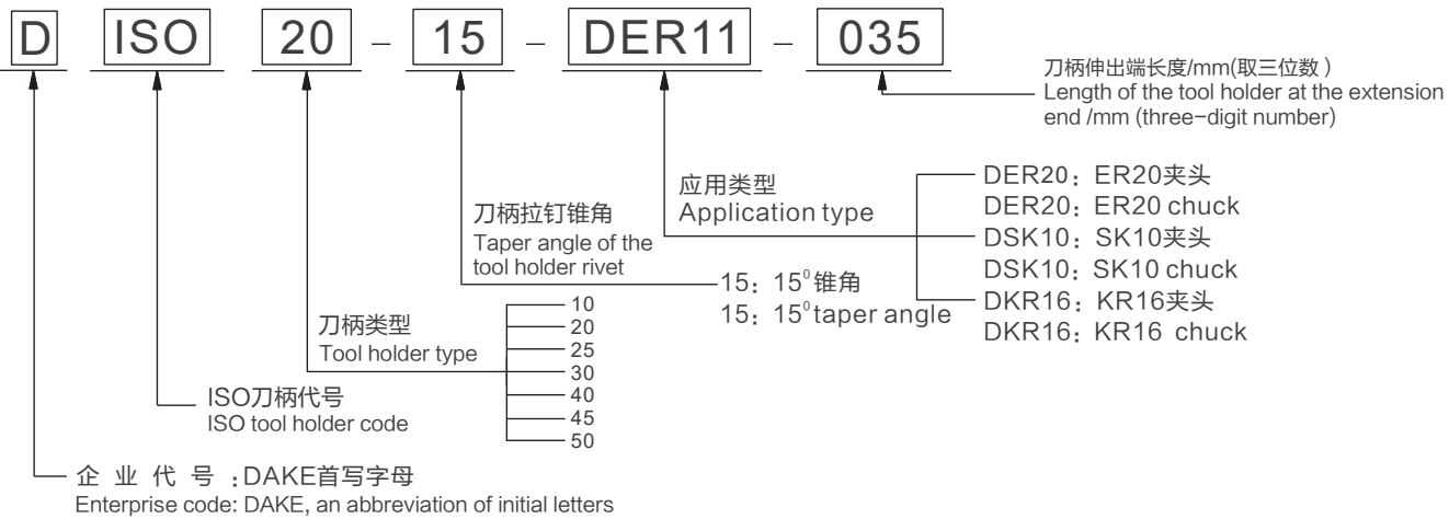
DISO-20-15-DER11-035 (命名示意图 Naming diagram)
