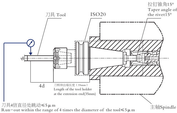
DISO-20-15-DER11-035 (装刀精度示意图 Tool installation precision diagram)
