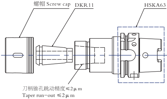
DHSCA63-DKR11-075 (命名示意图 Naming diagram)
