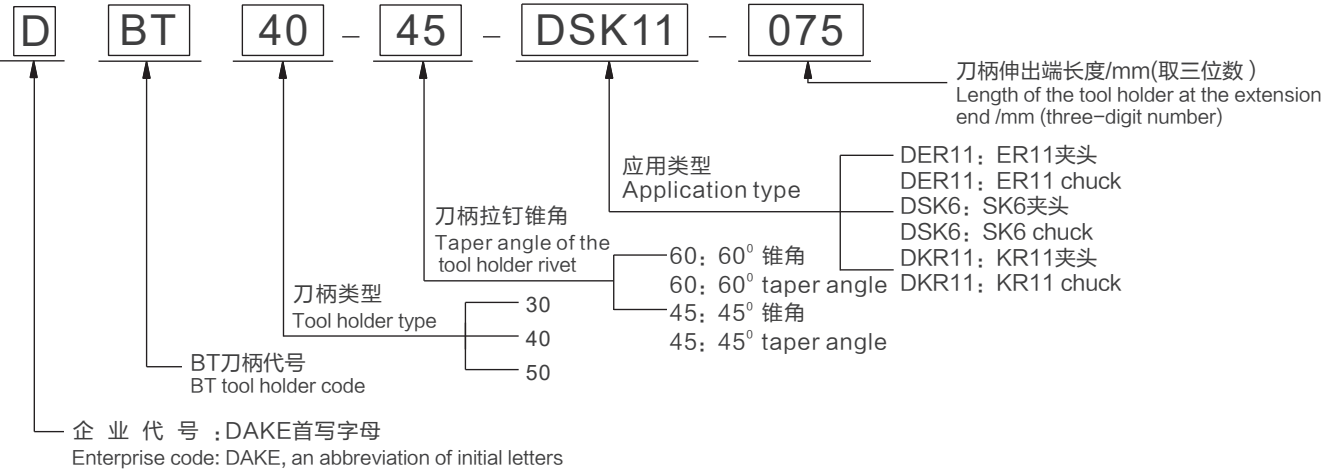
DBT40-45-DSK11-075 (命名示意图 Naming diagram)
