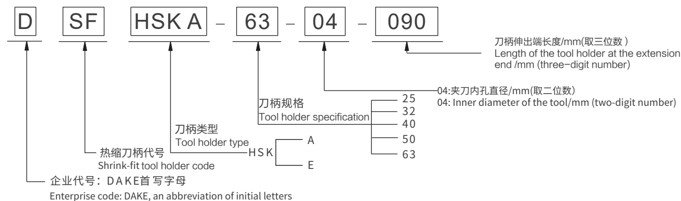
DSFHSA63-04-090 (示意图Schematic diagram)
