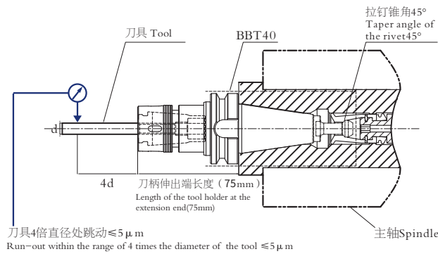
DBBT40-45-DSK11-075 (装刀精度示意图 Tool installation precision diagram)
