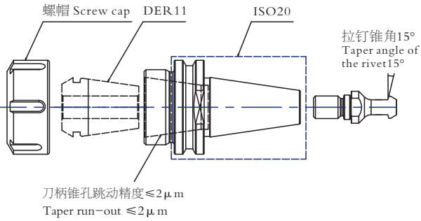
DISO-20-15-DER11-035 (命名示意图 Naming diagram)
