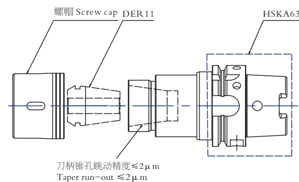
DHKA63-DER11-075 (命名示意图 Naming diagram)
