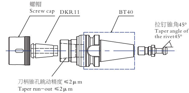
DBT40-45-DKR11-075 (命名示意图 Naming diagram)
