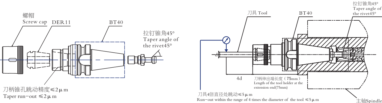
DBT40-45-DER11-075 (命名示意图 Naming diagram) DBT40-45-DER11-075 (装刀精度示意图 Tool installation precision diagram)
