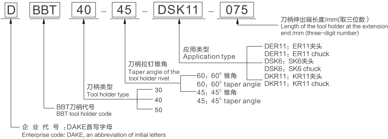
DBBT40-45-DSK11-075 (命名示意图 Naming diagram)
