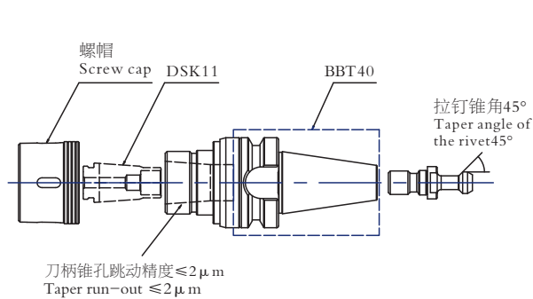
DBBT40-45-DSK11-075 (命名示意图 Naming diagram)
