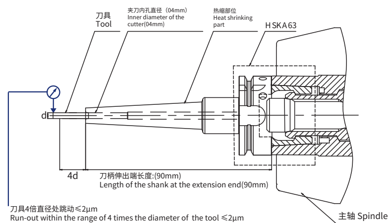
DSFHSA63-04-090 (示意图Schematic diagram)
